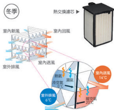
■ 熱交換濾芯內部 (示意機種：FV-47CZ1R)
