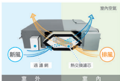
■ 熱交換原理說明 (示意機種：FY-E15PMAW)
