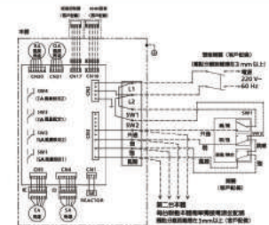
接線配置圖*1 FY-25ZY1W(220V)控制器另購
